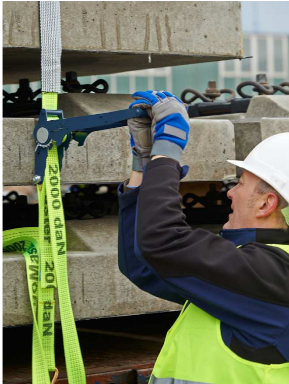
Abb. 3: Mit 720 daN erreicht die ErgoMaster eine ungewöhnlich hohe Vorspannkraft und ist damit bestens für das Niederzurren geeignet.
