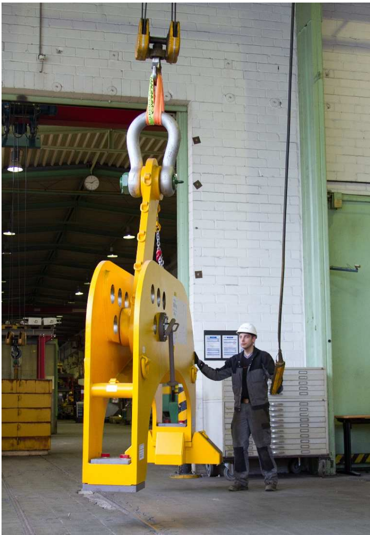
Abb. 1: Magnum-X short: Unverzichtbar bei kurzen Hubhöhen und äußerst kompakt durch Verwendung von Hochleistungsfasern.
